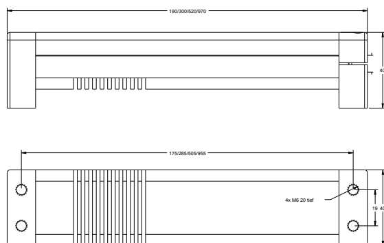
Serie ML-x-P ohne Fußblechset
