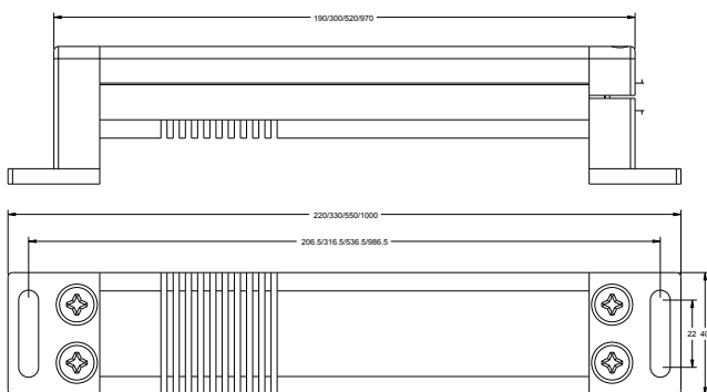
Serie ML-x-P mit Fußblechset
