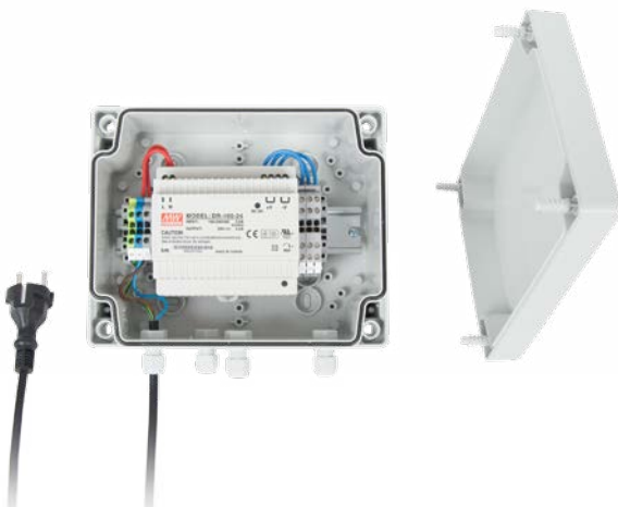
Stromversorgungsbox AL-PS-S
